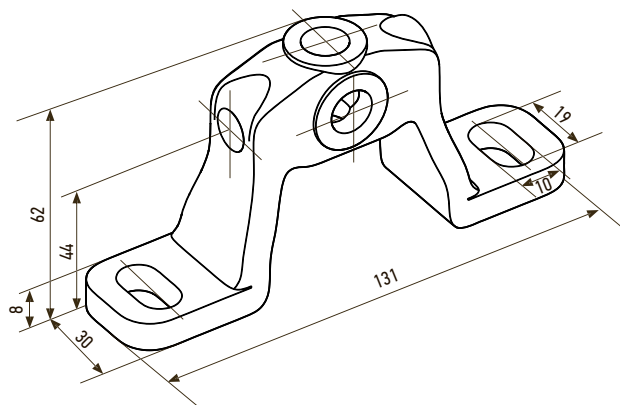
Кронштейн нижний
