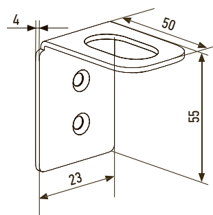
Кронштейн стеновой
