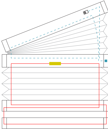
2 Schnurbohrungen/Cord boreholes/Passages de cordon 200-279 mm
