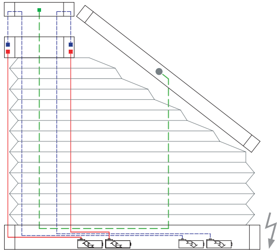
2 Drahtbohrungen/Wire boreholes/Passages de fil
