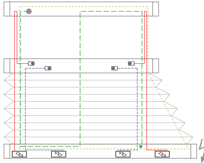
3 Drahtbohrungen/Wire boreholes/Passages de fil
