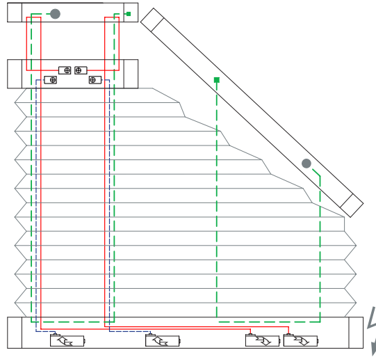
4 Drahtbohrungen/Wire boreholes/Passages de fil
