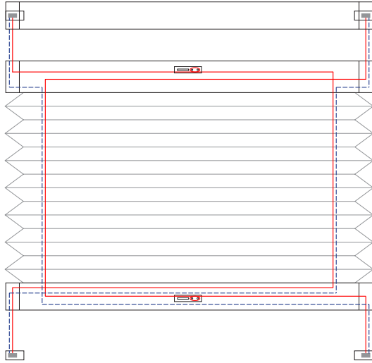
2 Schnurbohrungen/Cord boreholes/Passages de cordon 200-279 mm
