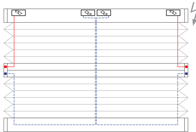
3 Schnurbohrungen/Cord boreholes/Passages de cordon
