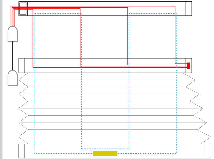
4 Schnurbohrungen/Cord boreholes/Passages de cordon
