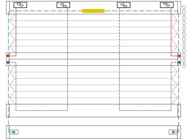
4 Schnurbohrungen/Cord boreholes/Passages de cordon
