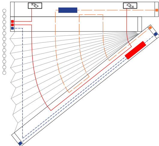
5 Schnurbohrungen/Cord boreholes/Passages de cordon
