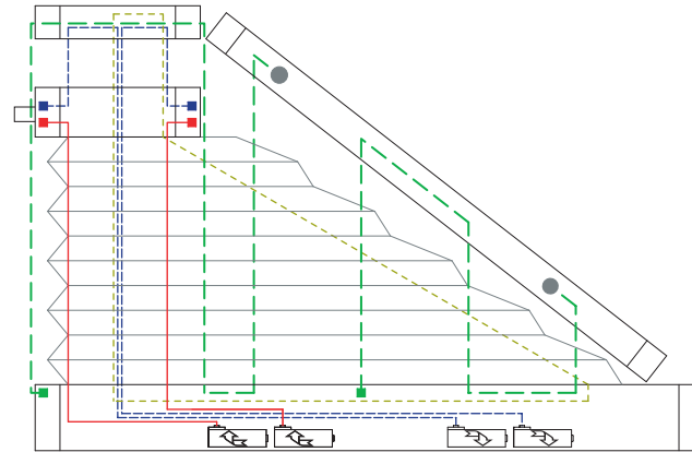
5 Drahtbohrungen/Wire boreholes/Passages de fil
