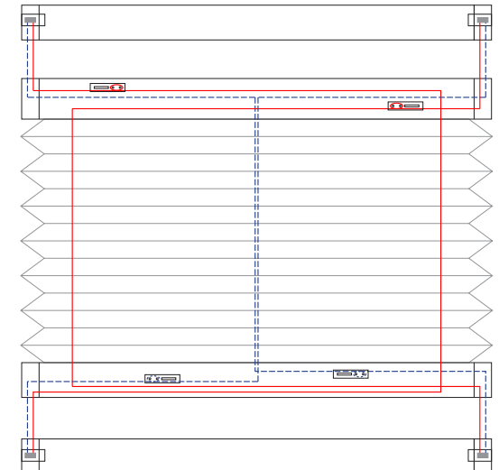
3 Schnurbohrungen/Cord boreholes/Passages de cordon
