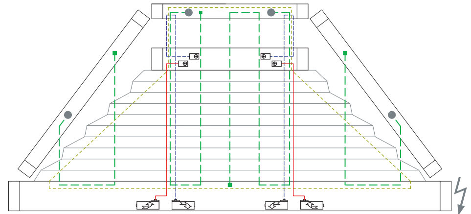
9 Drahtbohrungen/Wire boreholes/Passages de fil
