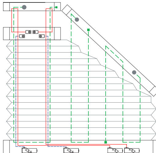
7 Drahtbohrungen/Wire boreholes/Passages de fil
