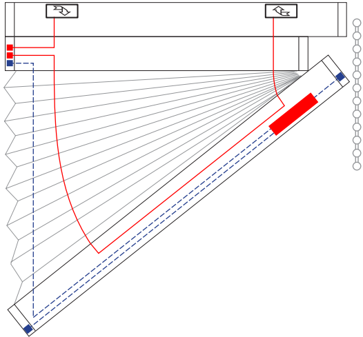
2 Schnurbohrungen/Cord boreholes/Passages de cordon
