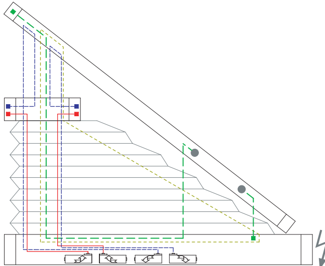
3 Drahtbohrungen/Wire boreholes/Passages de fil
