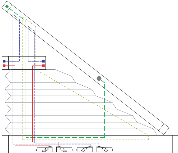
2 Drahtbohrungen/Wire boreholes/Passages de fil
