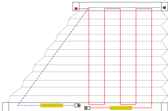
5 Schnurbohrungen/Cord boreholes/Passages de cordon
