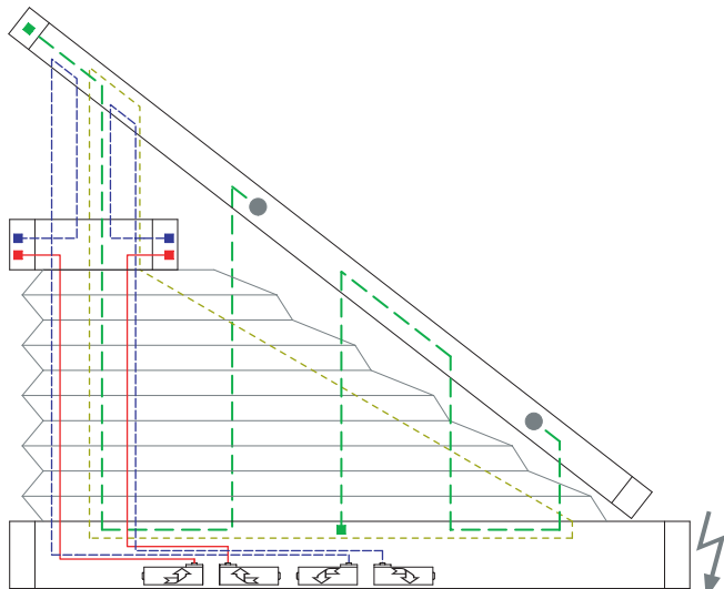
5 Drahtbohrungen/Wire boreholes/Passages de fil
