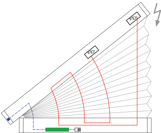
5 Schnurbohrungen/Cord boreholes/Passages de cordon
