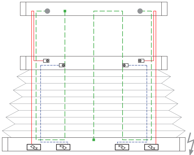
5 Drahtbohrungen/Wire boreholes/Passages de fil
