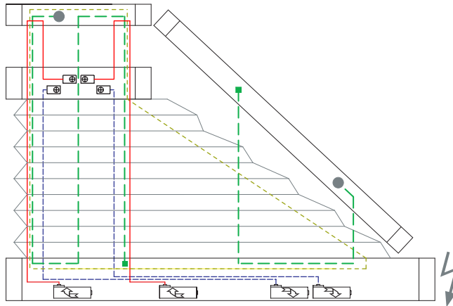
5 Drahtbohrungen/Wire boreholes/Passages de fil
