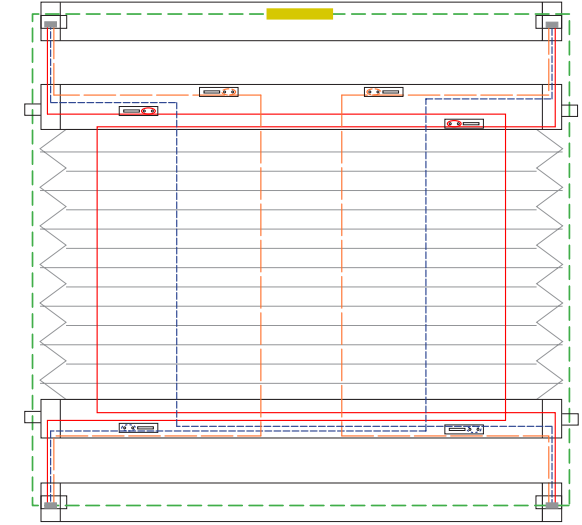
6 Schnurbohrungen/Cord boreholes/Passages de cordon
