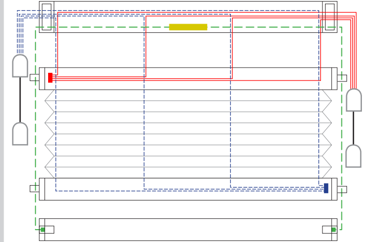
4 Schnurbohrungen/Cord boreholes/Passages de cordon
