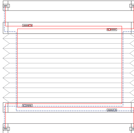
2 Schnurbohrungen/Cord boreholes/Passages de cordon ab/starting from/à partir de 280 mm
