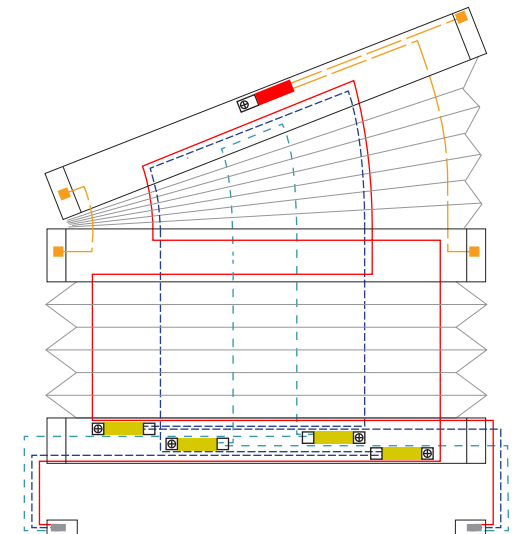
6 Schnurbohrungen/Cord boreholes/Passages de cordon
