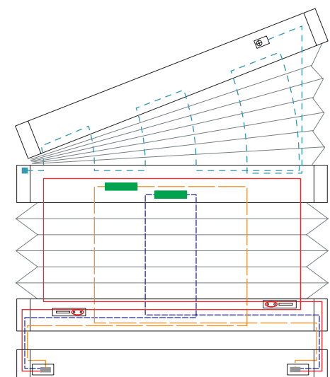
6 Schnurbohrungen/Cord boreholes/Passages de cordon
