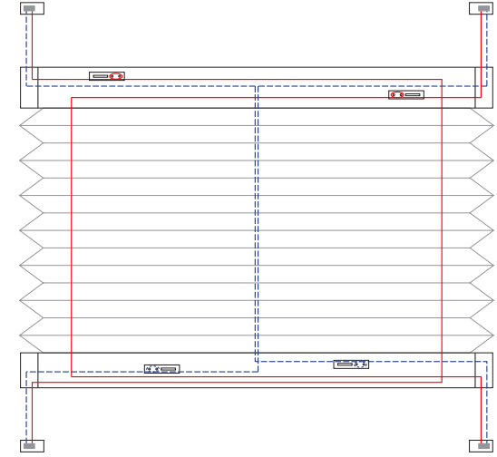
3 Schnurbohrungen/Cord boreholes/Passages de cordon
