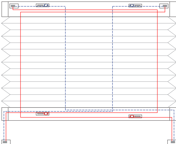
4 Schnurbohrungen/Cord boreholes/Passages de cordon
