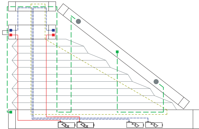
4 Drahtbohrungen/Wire boreholes/Passages de fil
