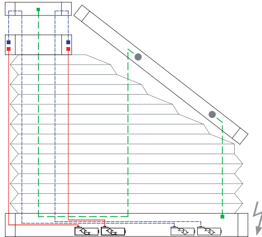
3 Drahtbohrungen/Wire boreholes/Passages de fil
