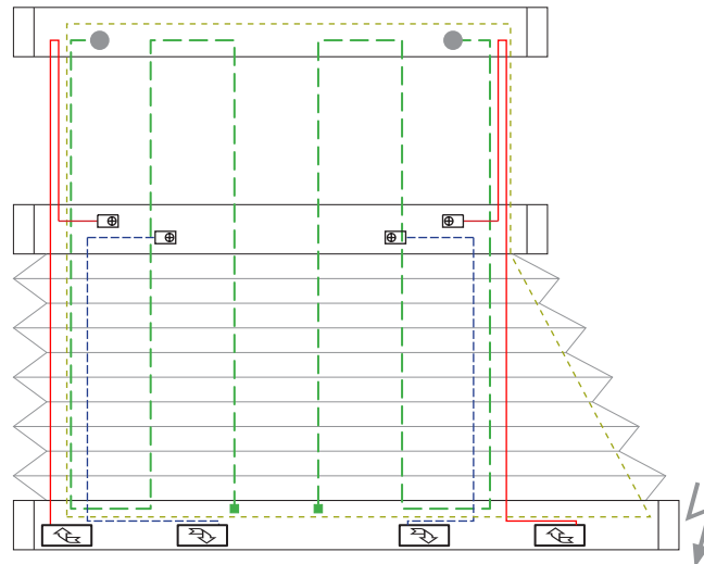
6 Drahtbohrungen/Wire boreholes/Passages de fil
