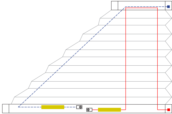
2 Schnurbohrungen/Cord boreholes/Passages de cordon
