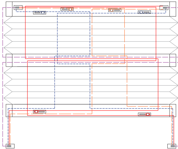
5 Schnurbohrungen/Cord boreholes/Passages de cordon
