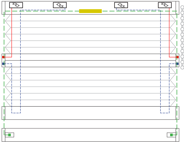
2 Schnurbohrungen/Cord boreholes/Passages de cordon
