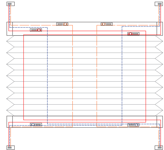
6 Schnurbohrungen/Cord boreholes/Passages de cordon
