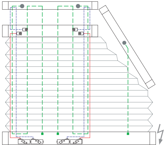
7 Drahtbohrungen/Wire boreholes/Passages de fil
