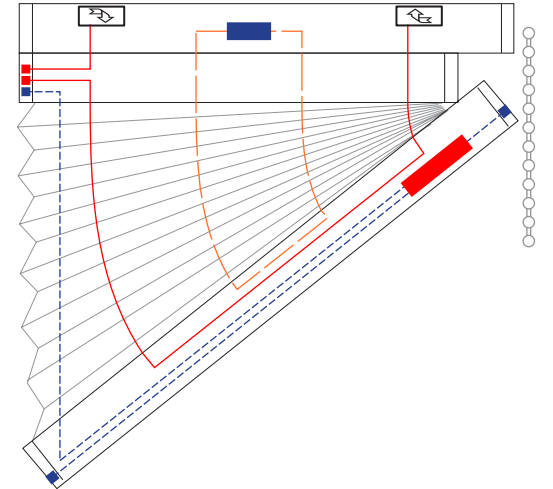
4 Schnurbohrungen/Cord boreholes/Passages de cordon
