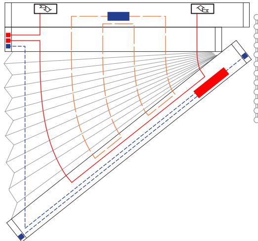
6 Schnurbohrungen/Cord boreholes/Passages de cordon
