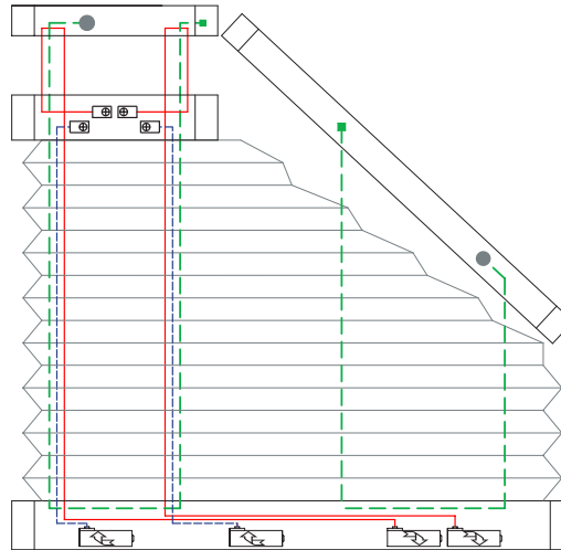
4 Drahtbohrungen/Wire boreholes/Passages de fil
