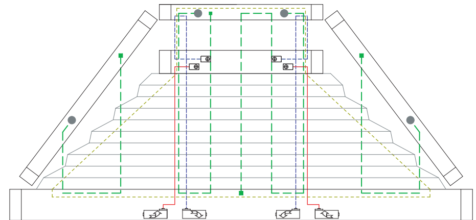
9 Drahtbohrungen/Wire boreholes/Passages de fil
