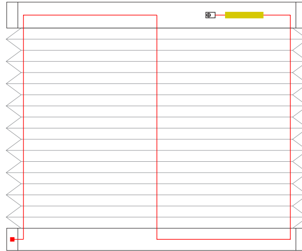
3 Schnurbohrungen/Cord boreholes/Passages de cordon
