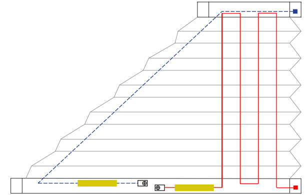
4 Schnurbohrungen/Cord boreholes/Passages de cordon
