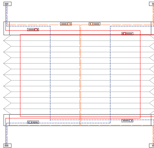
5 Schnurbohrungen/Cord boreholes/Passages de cordon
