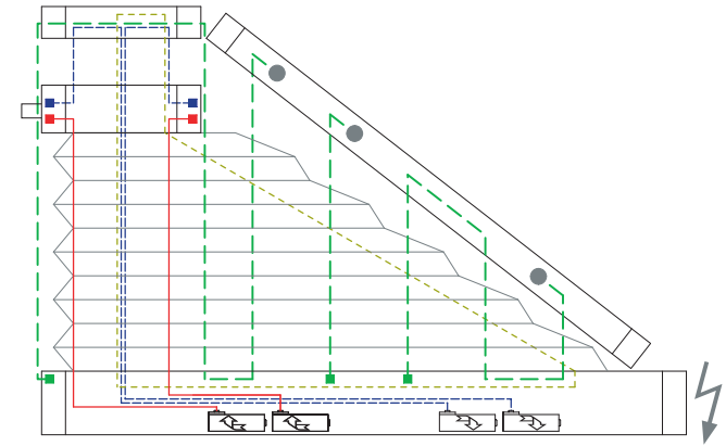
6 Drahtbohrungen/Wire boreholes/Passages de fil
