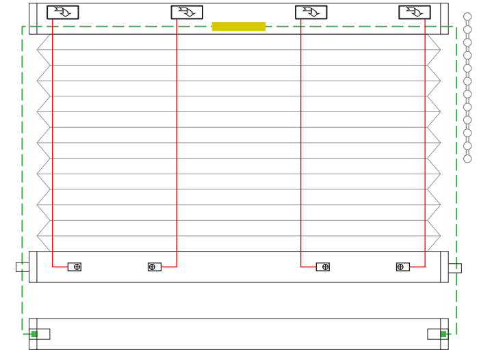
4 Schnurbohrungen/Cord boreholes/Passages de cordon
