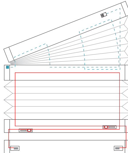
2 Schnurbohrungen/Cord boreholes/Passages de cordon ab/starting from/à partir de 280 mm
