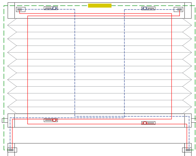
4 Schnurbohrungen/Cord boreholes/Passages de cordon
