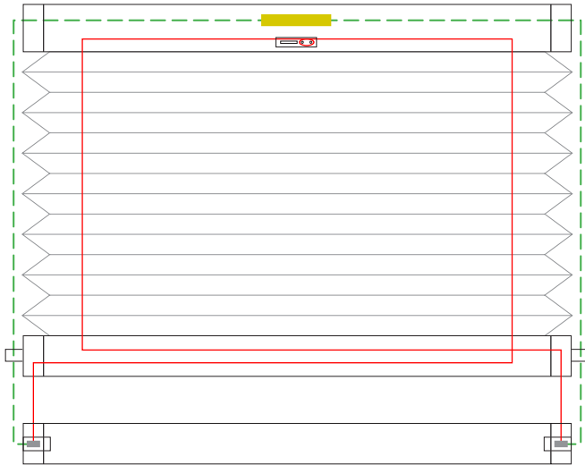
2 Schnurbohrungen/Cord boreholes/Passages de cordon 200-279 mm
