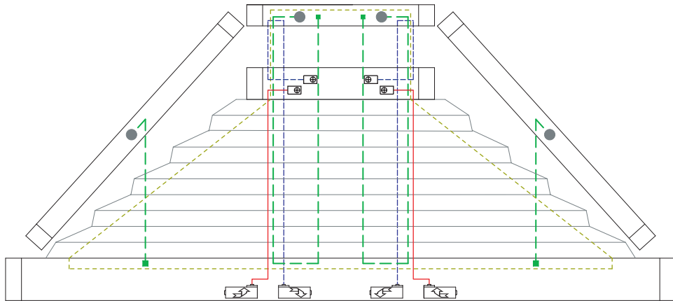
6 Drahtbohrungen/Wire boreholes/Passages de fil
