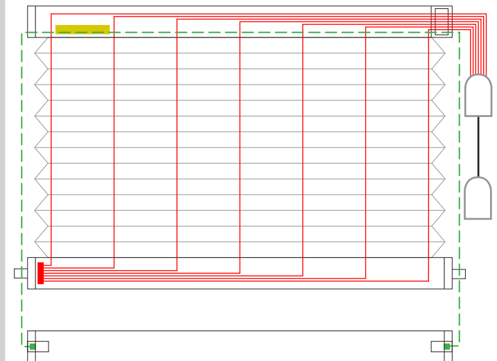
7 Schnurbohrungen/Cord boreholes/Passages de cordon
