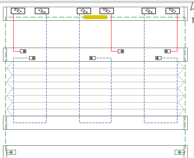
6 Schnurbohrungen/Cord boreholes/Passages de cordon
