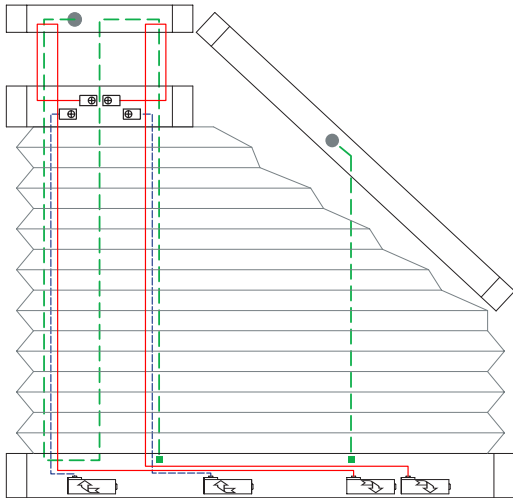
4 Drahtbohrungen/Wire boreholes/Passages de fil
