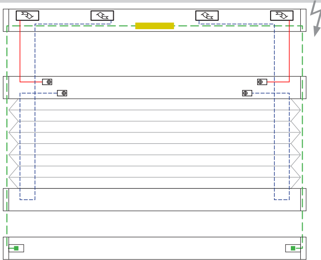
2 Schnurbohrungen/Cord boreholes/Passages de cordon
