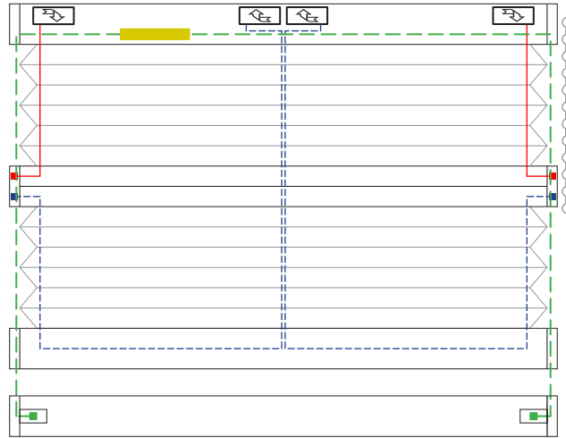
3 Schnurbohrungen/Cord boreholes/Passages de cordon
