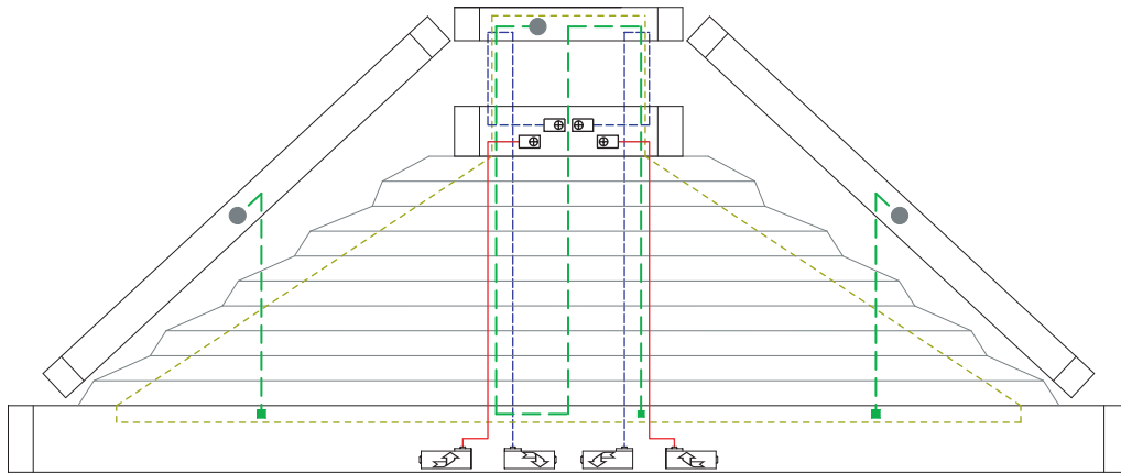
5 Drahtbohrungen/Wire boreholes/Passages de fil
