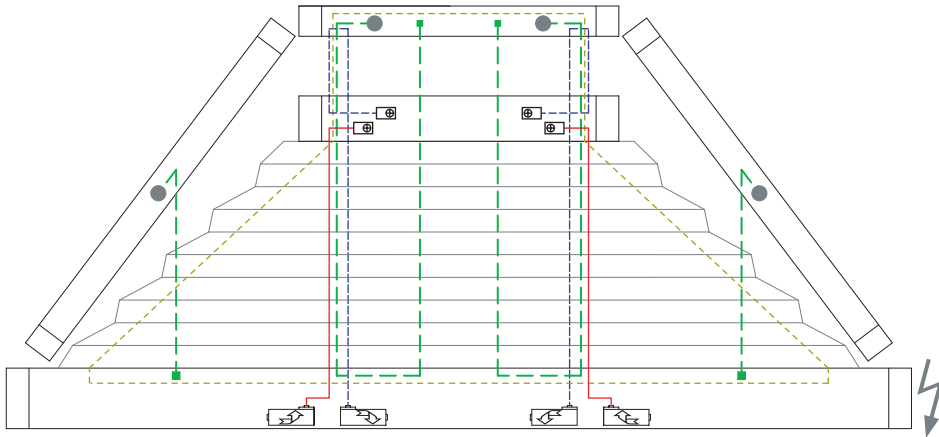
6 Drahtbohrungen/Wire boreholes/Passages de fil
