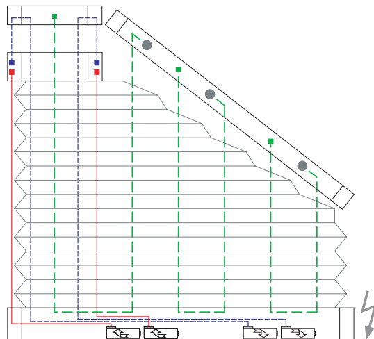
6 Drahtbohrungen/Wire boreholes/Passages de fil
