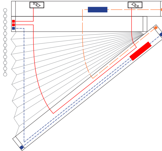
3 Schnurbohrungen/Cord boreholes/Passages de cordon
