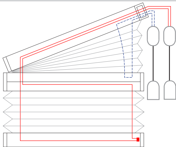
2 Schnurbohrungen/Cord boreholes/Passages de cordon
