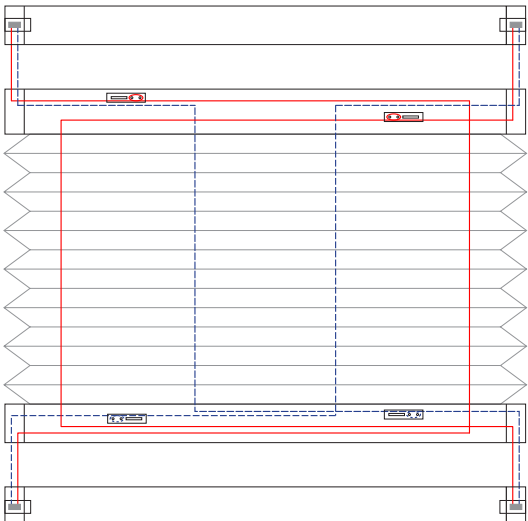
4 Schnurbohrungen/Cord boreholes/Passages de cordon
