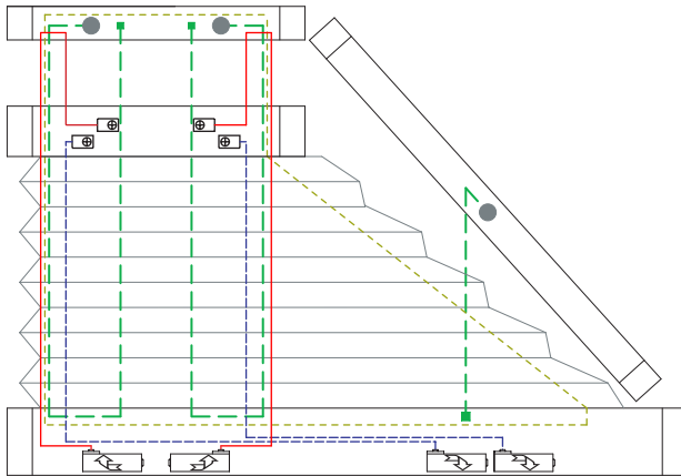
5 Drahtbohrungen/Wire boreholes/Passages de fil
