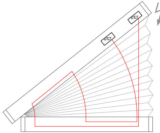
3 Schnurbohrungen/Cord boreholes/Passages de cordon
