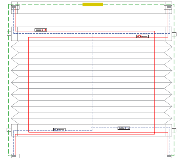
3 Schnurbohrungen/Cord boreholes/Passages de cordon
