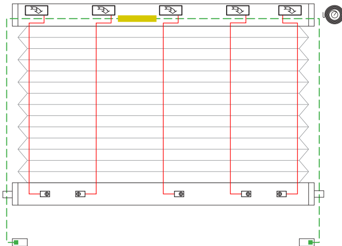
5 Schnurbohrungen/Cord boreholes/Passages de cordon
