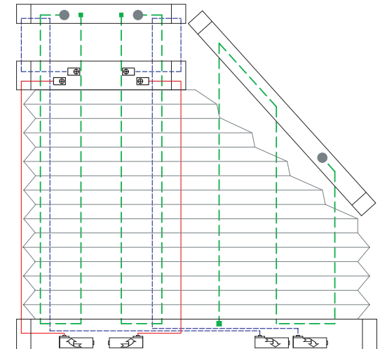
7 Drahtbohrungen/Wire boreholes/Passages de fil
