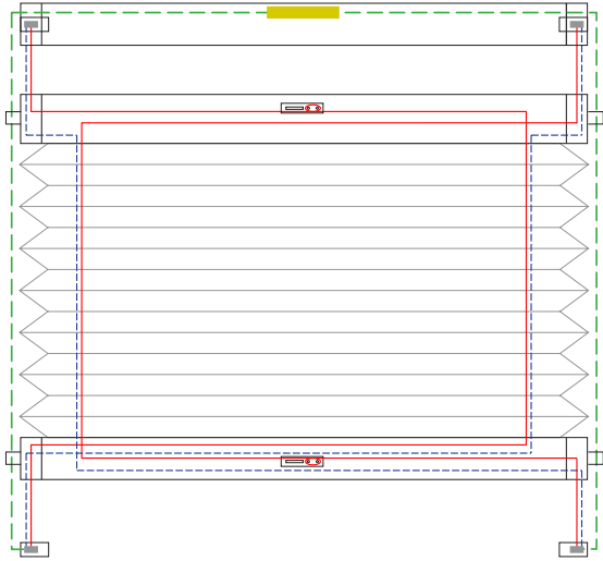
2 Schnurbohrungen/Cord boreholes/Passages de cordon 200-279 mm
