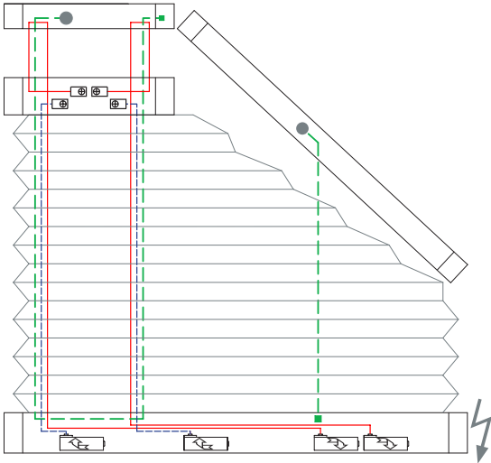
3 Drahtbohrungen/Wire boreholes/Passages de fil
