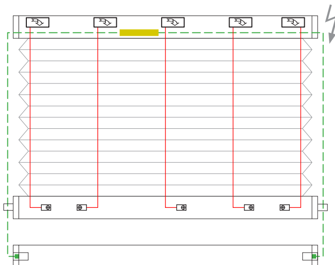
5 Schnurbohrungen/Cord boreholes/Passages de cordon
