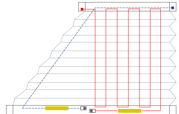
7 Schnurbohrungen/Cord boreholes/Passages de cordon
