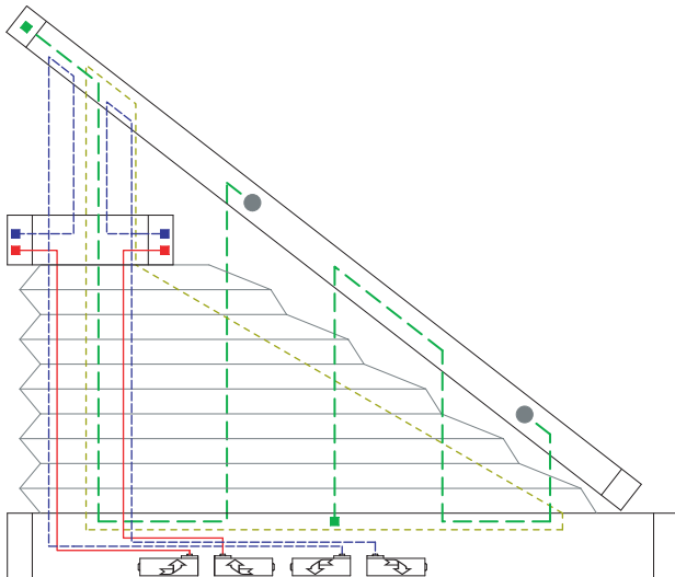
5 Drahtbohrungen/Wire boreholes/Passages de fil
