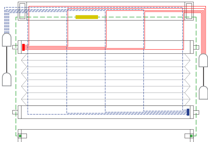
5 Schnurbohrungen/Cord boreholes/Passages de cordon
