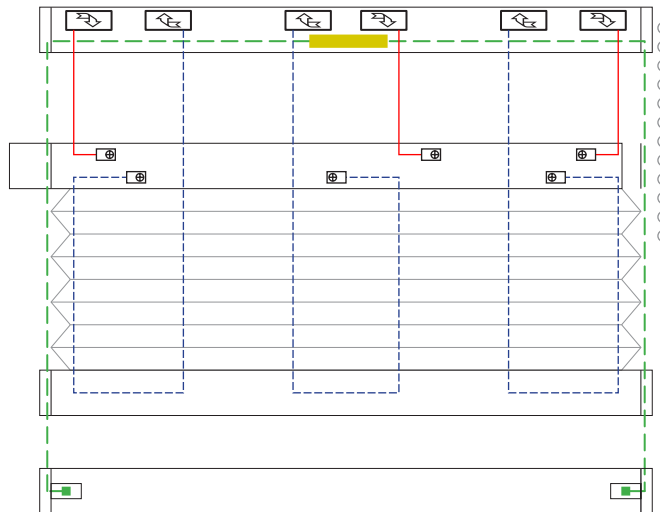
6 Schnurbohrungen/Cord boreholes/Passages de cordon
