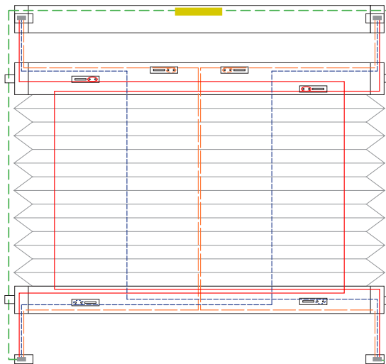
5 Schnurbohrungen/Cord boreholes/Passages de cordon
