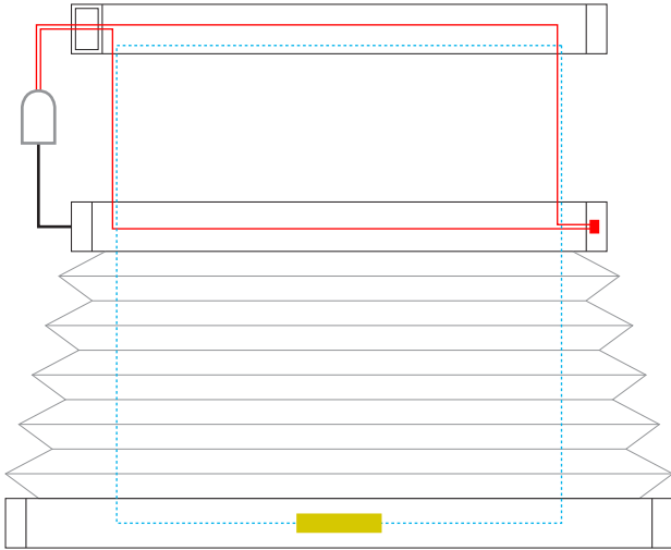
2 Schnurbohrungen/Cord boreholes/Passages de cordon
