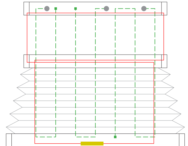
7 Drahtbohrungen/Wire boreholes/Passages de fil
