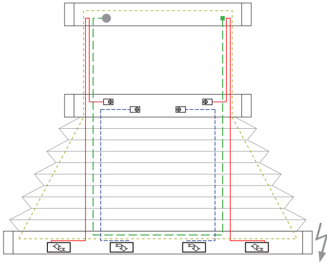
2 Drahtbohrungen/Wire boreholes/Passages de fil
