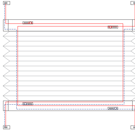
2 Schnurbohrungen/Cord boreholes/Passages de cordon ab/starting from/à partir de 280 mm
