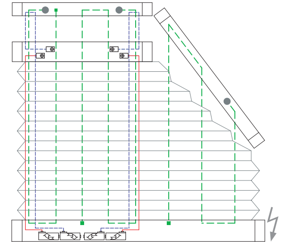
8 Drahtbohrungen/Wire boreholes/Passages de fil
