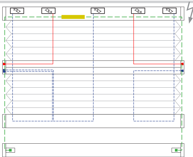
5 Schnurbohrungen/Cord boreholes/Passages de cordon
