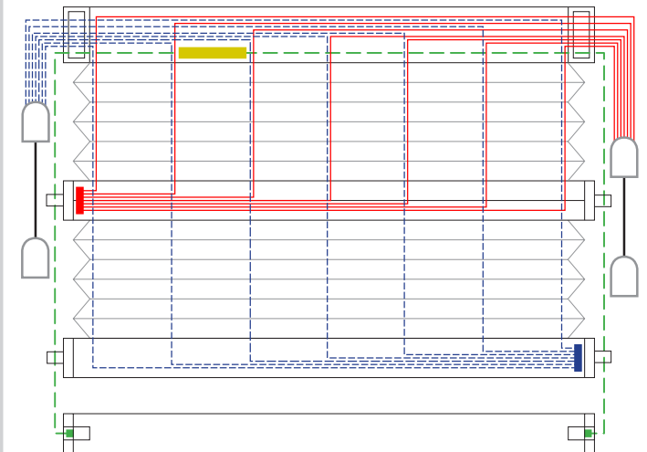
7 Schnurbohrungen/Cord boreholes/Passages de cordon
