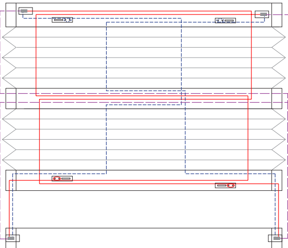
4 Schnurbohrungen/Cord boreholes/Passages de cordon
