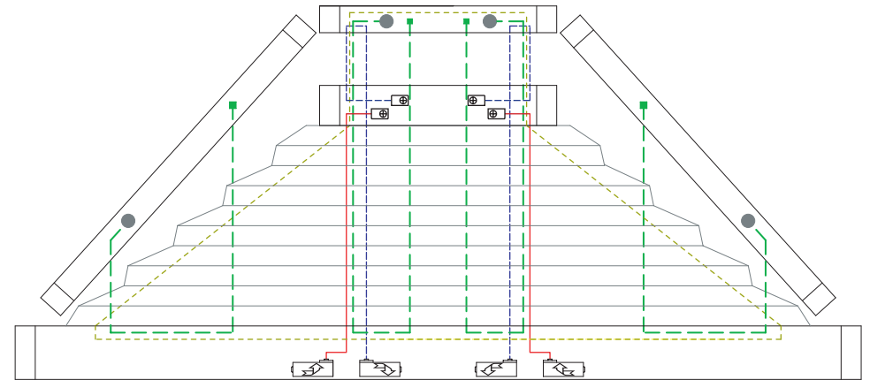
8 Drahtbohrungen/Wire boreholes/Passages de fil
