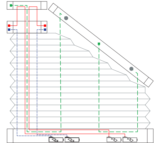
4 Drahtbohrungen/Wire boreholes/Passages de fil
