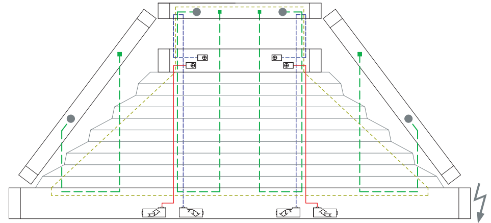
8 Drahtbohrungen/Wire boreholes/Passages de fil
