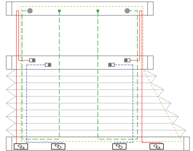
4 Drahtbohrungen/Wire boreholes/Passages de fil
