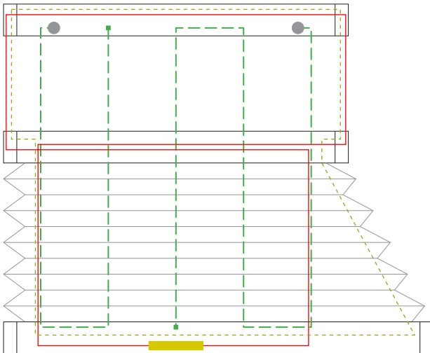
5 Drahtbohrungen/Wire boreholes/Passages de fil
