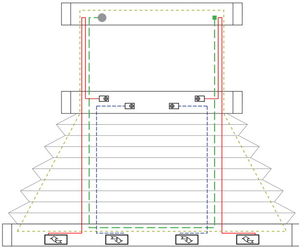
2 Drahtbohrungen/Wire boreholes/Passages de fil
