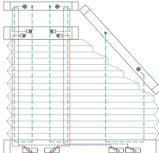
6 Drahtbohrungen/Wire boreholes/Passages de fil
