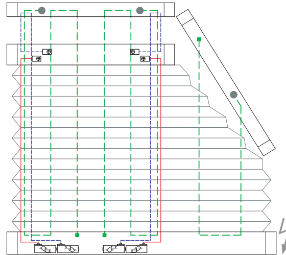
8 Drahtbohrungen/Wire boreholes/Passages de fil
