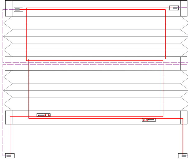
2 Schnurbohrungen/Cord boreholes/Passages de cordon ab/starting from/à partir de 280 mm
