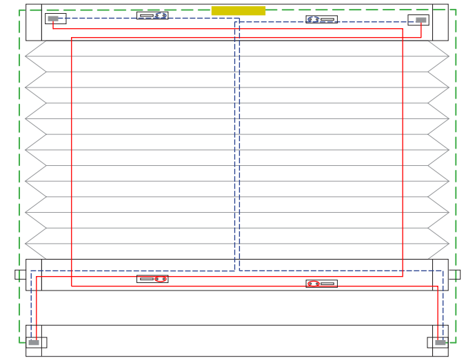
3 Schnurbohrungen/Cord boreholes/Passages de cordon
