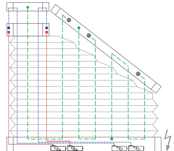
7 Drahtbohrungen/Wire boreholes/Passages de fil
