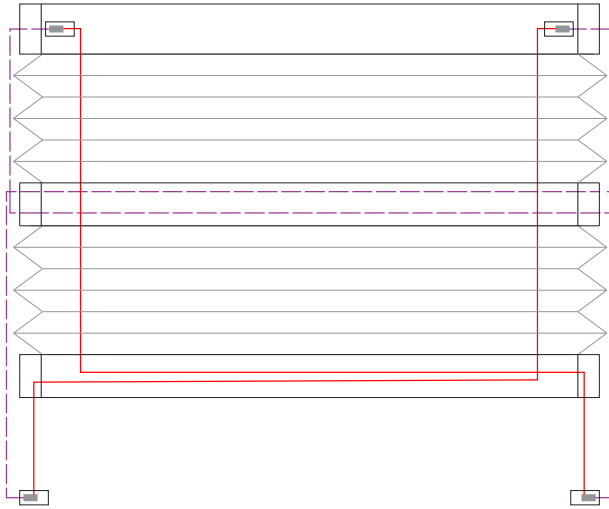
2 Schnurbohrungen/Cord boreholes/Passages de cordon 200-279 mm
