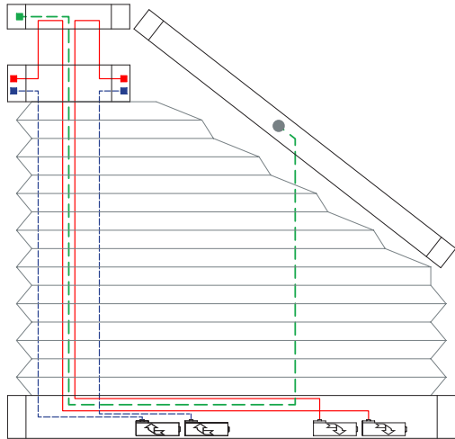
2 Drahtbohrungen/Wire boreholes/Passages de fil
