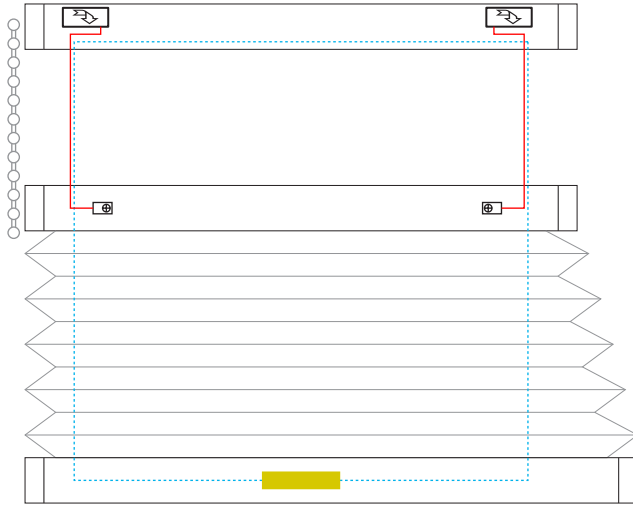
2 Schnurbohrungen/Cord boreholes/Passages de cordon
