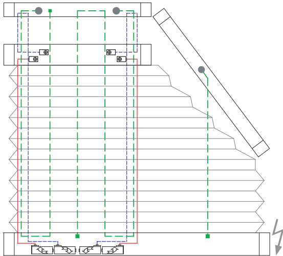
6 Drahtbohrungen/Wire boreholes/Passages de fil
