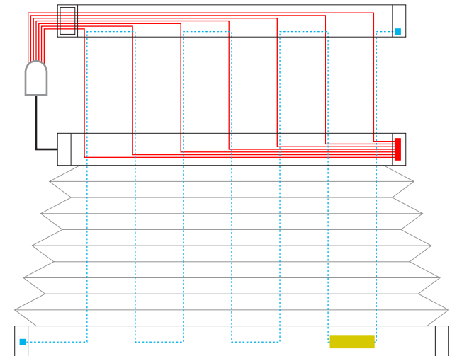
7 Schnurbohrungen/Cord boreholes/Passages de cordon
