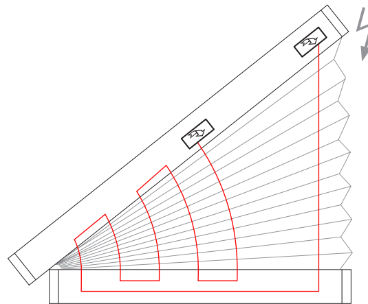
6 Schnurbohrungen/Cord boreholes/Passages de cordon
