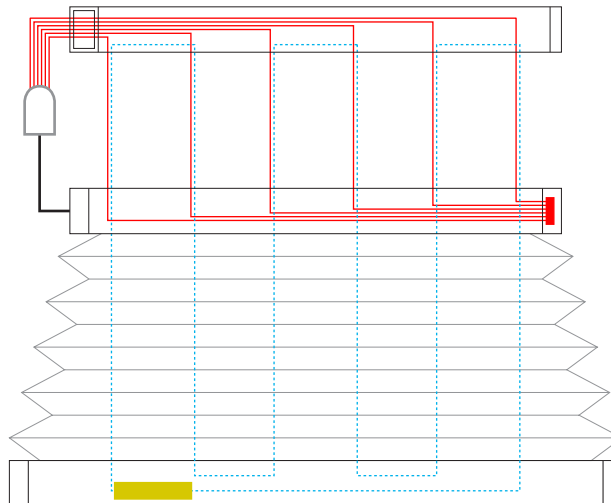
6 Schnurbohrungen/Cord boreholes/Passages de cordon
