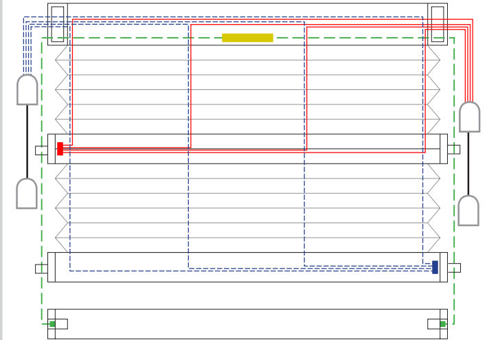
4 Schnurbohrungen/Cord boreholes/Passages de cordon
