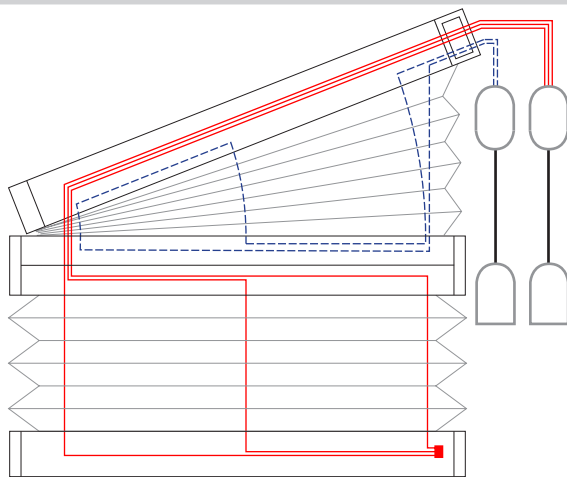
3 Schnurbohrungen/Cord boreholes/Passages de cordon
