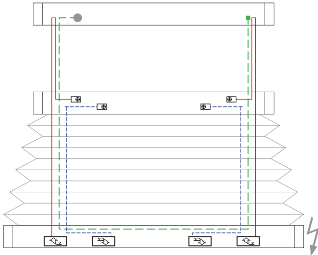
2 Drahtbohrungen/Wire boreholes/Passages de fil
