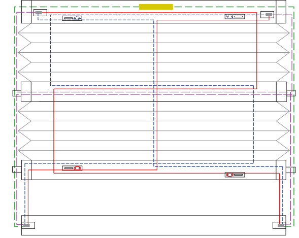
3 Schnurbohrungen/Cord boreholes/Passages de cordon
