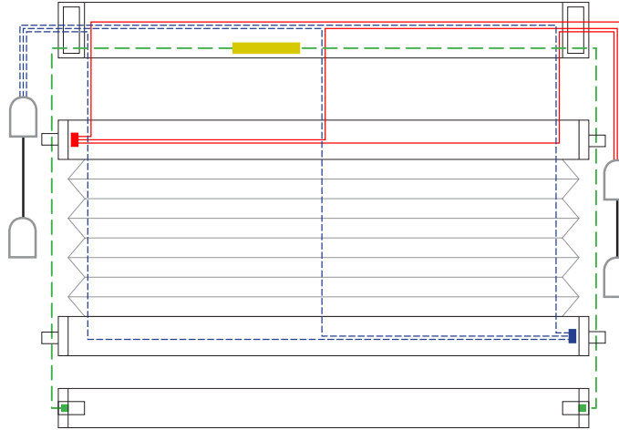
3 Schnurbohrungen/Cord boreholes/Passages de cordon
