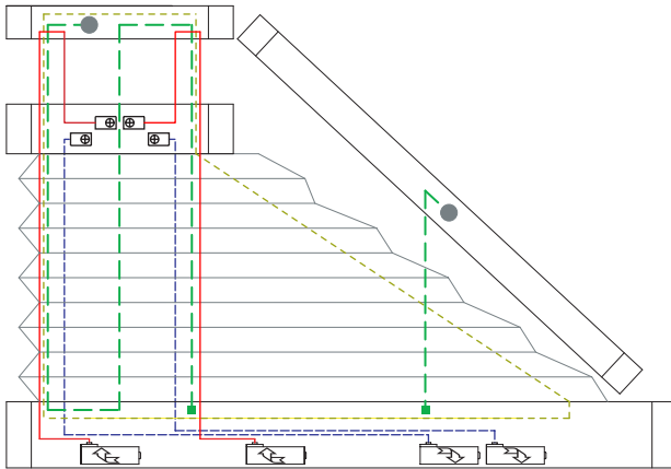
4 Drahtbohrungen/Wire boreholes/Passages de fil
