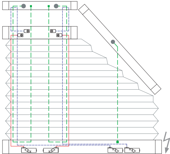
5 Drahtbohrungen/Wire boreholes/Passages de fil
