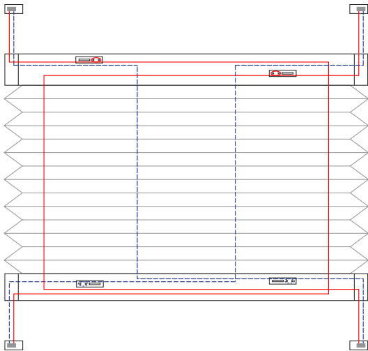
4 Schnurbohrungen/Cord boreholes/Passages de cordon
