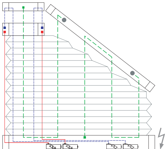
5 Drahtbohrungen/Wire boreholes/Passages de fil
