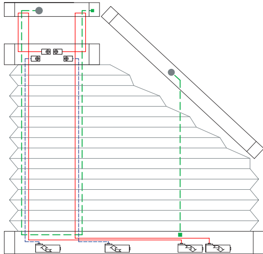
3 Drahtbohrungen/Wire boreholes/Passages de fil
